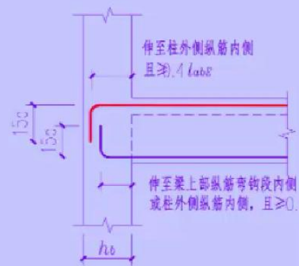
KL端部纵向钢筋弯锚构造
